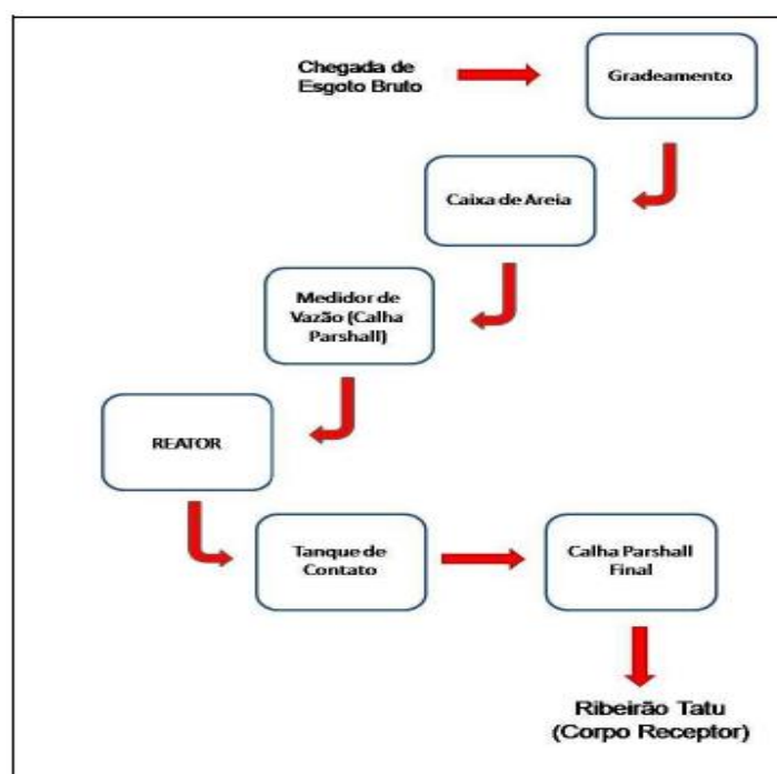
Figura 28. Sistema de Tratamento de Esgoto proposto para o município de Cordeirópolis – SP.
