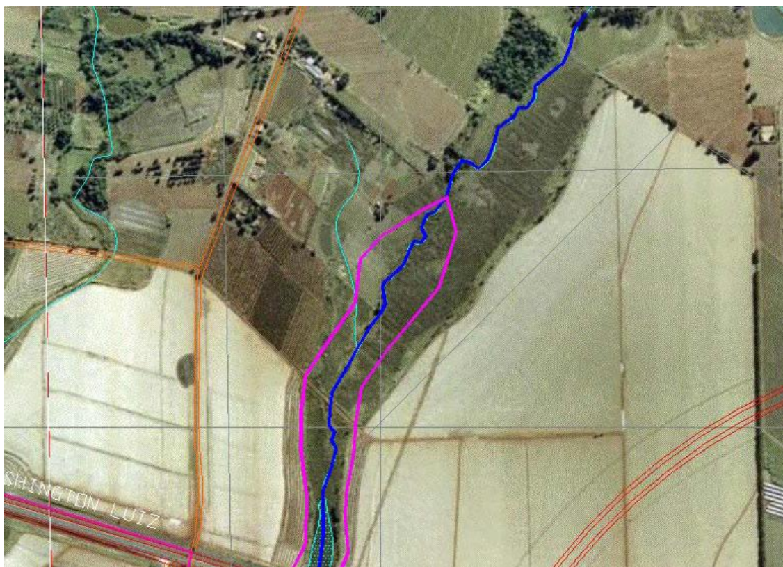
Figura 40. Nova Represa Santa Marina projetada pela empresa MKMBr Engenharia Ambiental.
