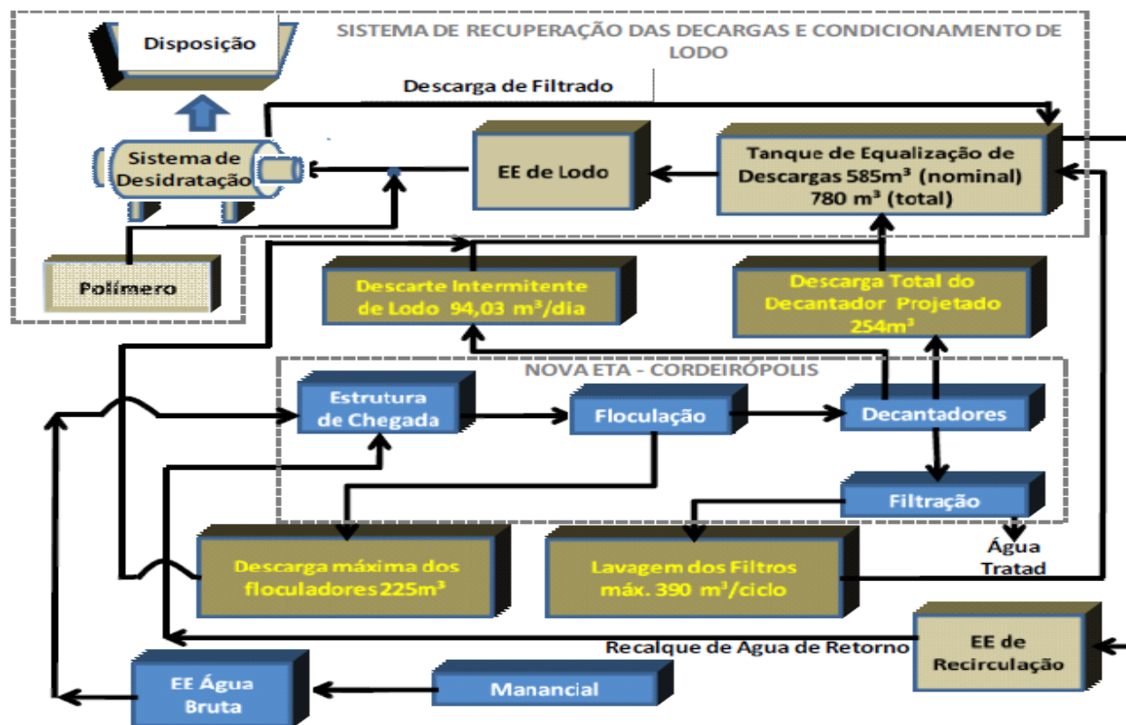
Figura 38. Fluxograma do processo da nova ETA extraído do projeto executivo elaborado pela empresa PROESPLAN Engenharia LTDA.
